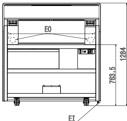
Oldalnézet
